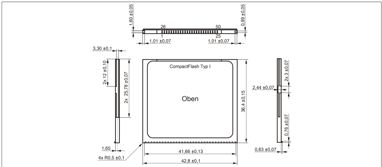
Abbildung 1: Abmessungen CompactFlash-Karte Typ I
