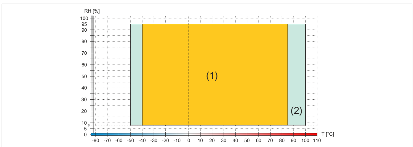
Abbildung 2: Temperatur Luftfeuchtediagramm Compact Flash Karten 0CFCRD.xxxxE.01
