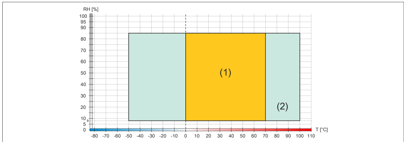
Abbildung 3: 5CFCRD.xxxx-06 - Temperatur Luftfeuchtediagramm CompactFlash-Karten
