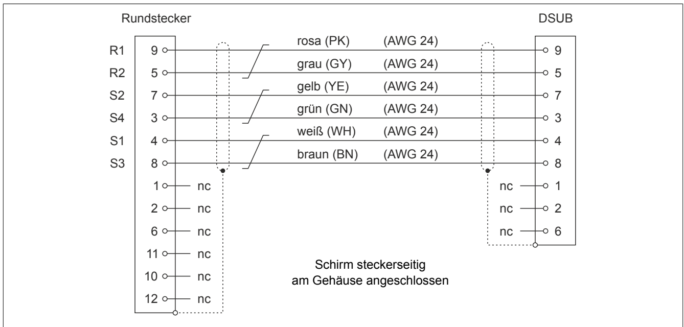
Abbildung 1: Kabelplan Resolverkabel
