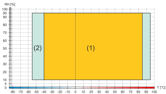
Abbildung 2: 5AC901.CSSD-06 - Temperatur-Luftfeuchte-Diagramm - ab Rev. D0
