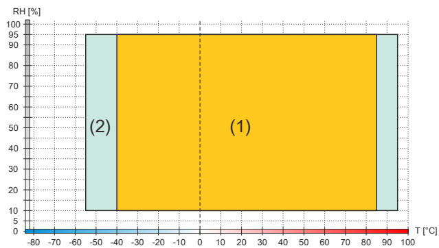
Abbildung 1: 5AC901.CSSD-05 - Temperatur-Luftfeuchte-Diagramm - ab Rev. F0
